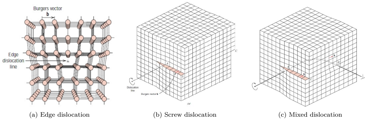
Figura 1.3: Tipos de dislocaciones.
