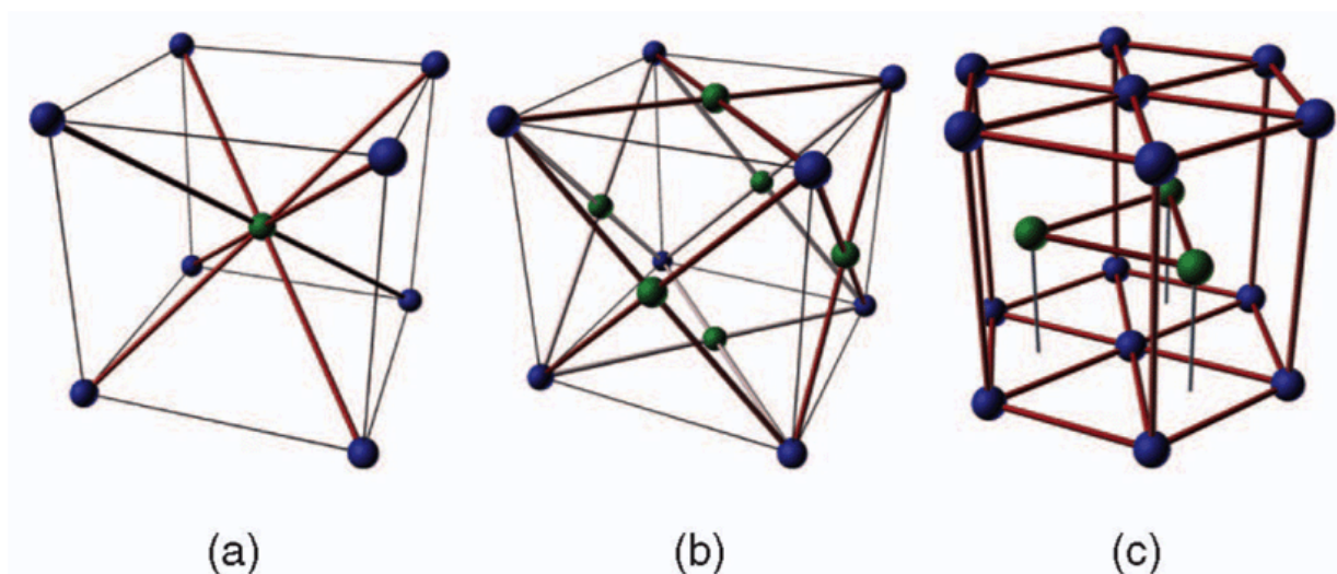
Figura 1.1: Ejemplos esquemáticos de las redes BCC (a), FCC (b), y HCP (c).
