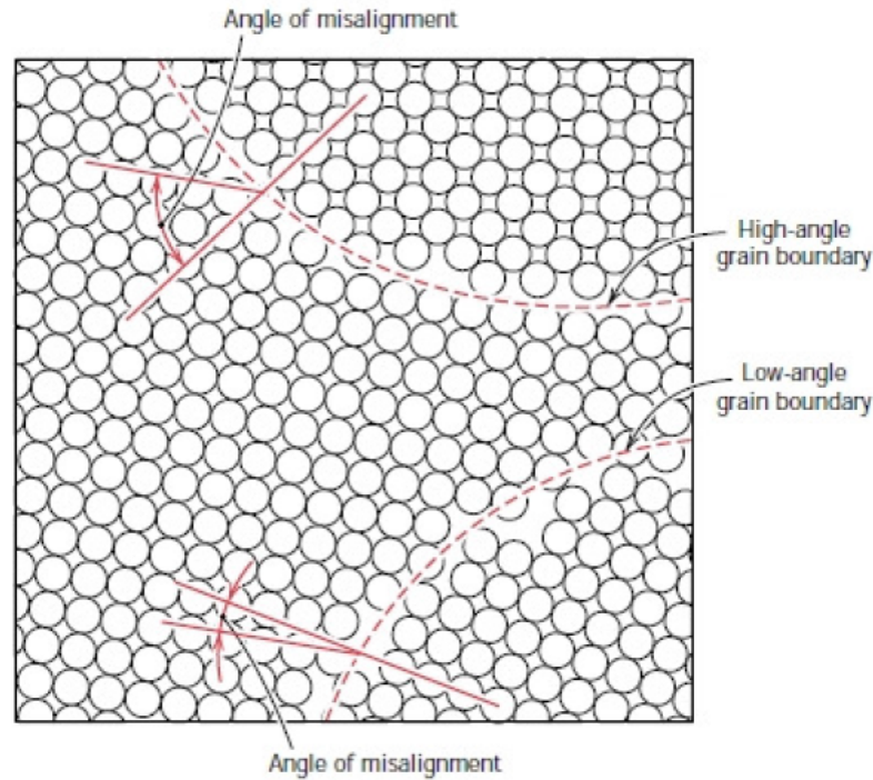
Figura 1.5: Bordes de grano de alto y bajo ángulo de desalineación.
