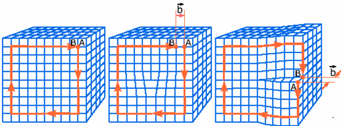
Figura 1.4: Vector de Burgers para dislocaciones lineales y de tornillo.
