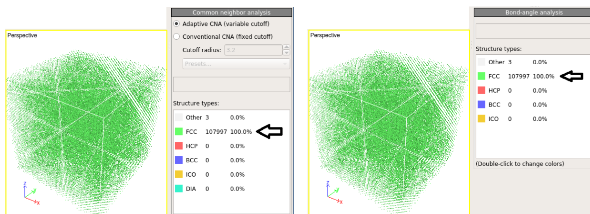
Figura 2.2: Resultados de los estudios tipo Common neighbor analysis (CNA) y Bond-angle analysis .
