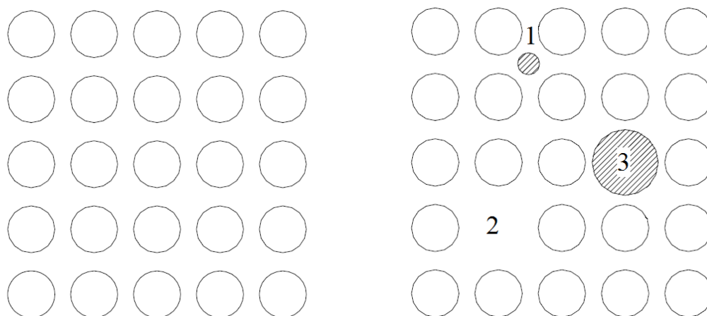
Figura 1.2: Defectos puntuales (derecha) sobre una estructura perfecta (izquierda): intersticial (1), vacante (2) y sustitución (3).
