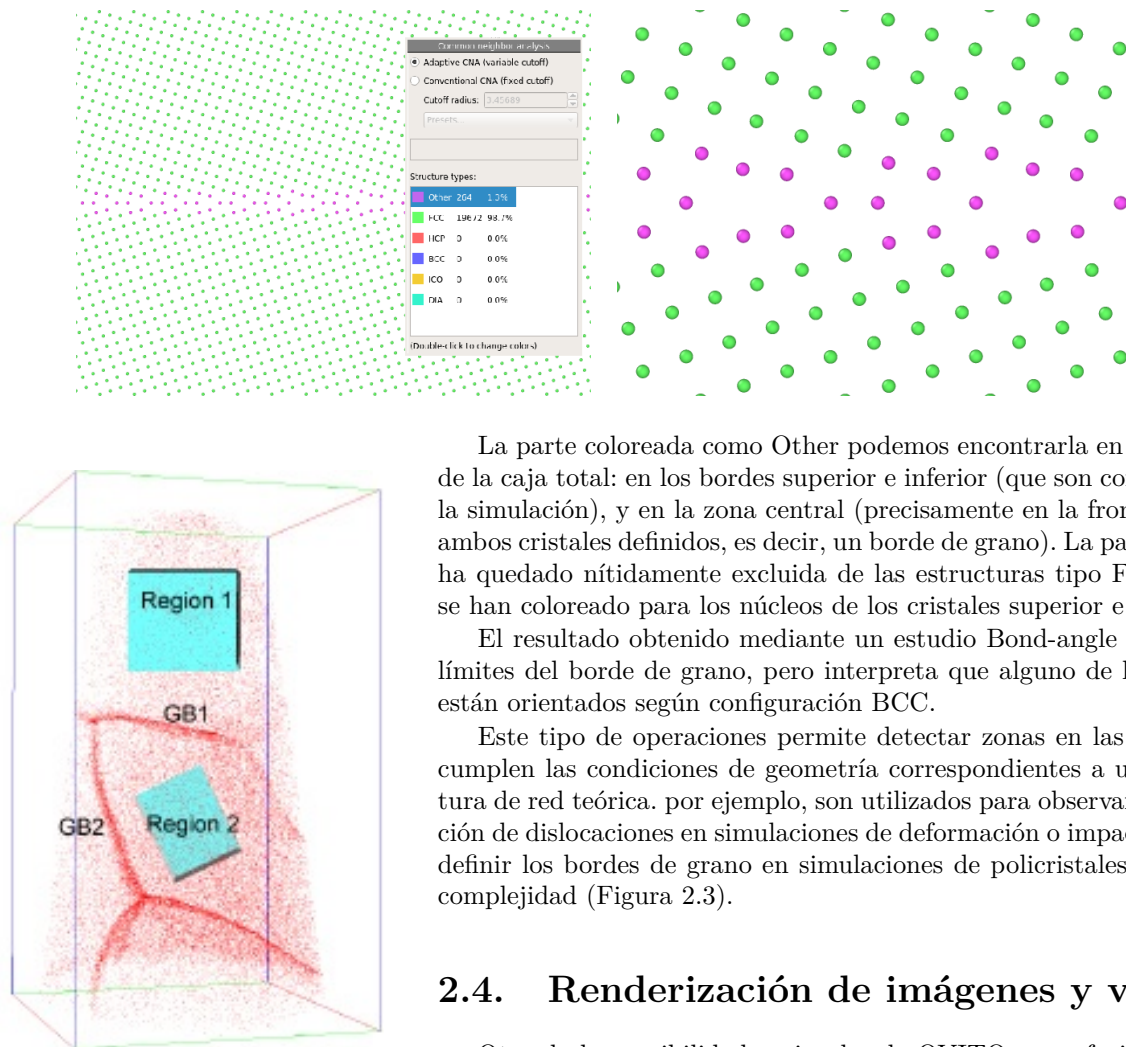
Figura 2.3: Detección de un borde de grano durante la simulación de un hilo superconductor ( M. J. R. Sandim et al, 2013, Supercond. Sci. Technol. 26 055008 )
