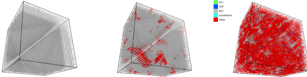
Figura 1.6: Evolución de una estructura BCC a través de CNA.
