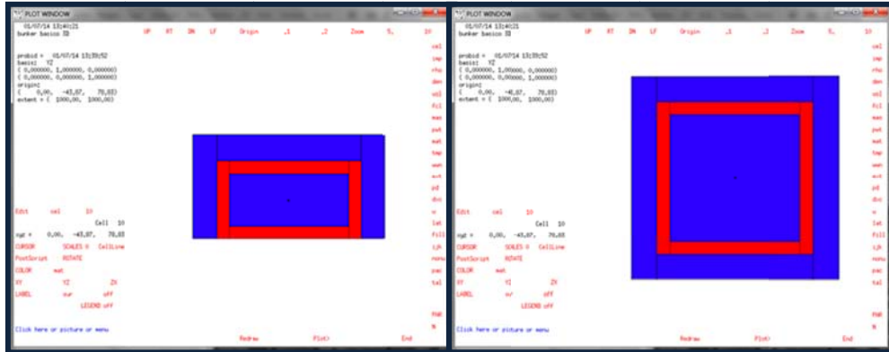
Figura 6. Visualización de la geometría del búnker diseñado para la práctica con los alumnos mediante el visor de MCNPX.
